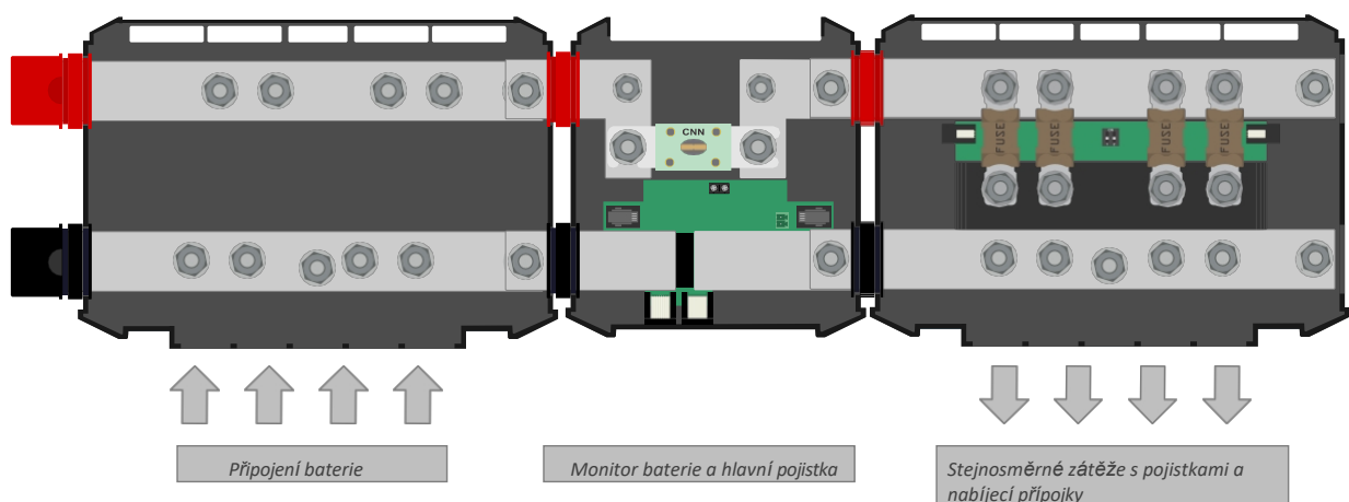
Obrázek 2. Příklad propojených modulů Lynx bez krytů (Lynx Shunt VE.Can)
