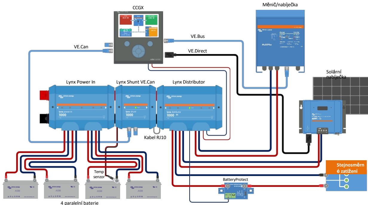
Systém s bočником Lynx VE.Can, olověnými akumulátory, bočником Lynx VE.Can a rozdělovačem Lynx.
