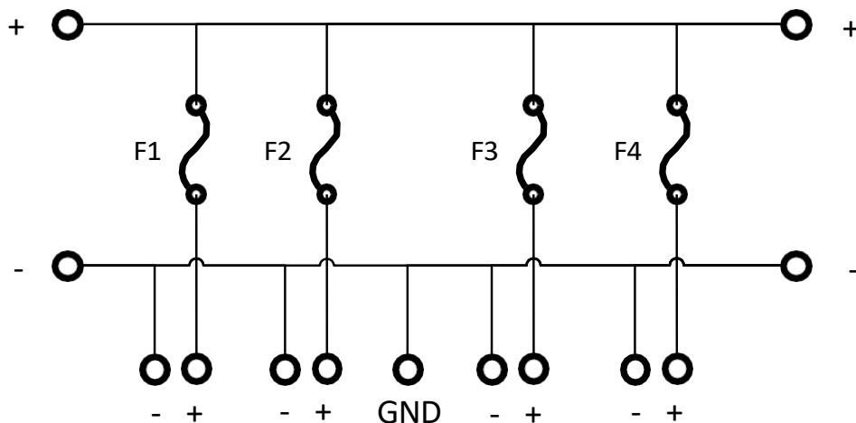
Schéma vnitřního zapojení rozdělovače Lynx
