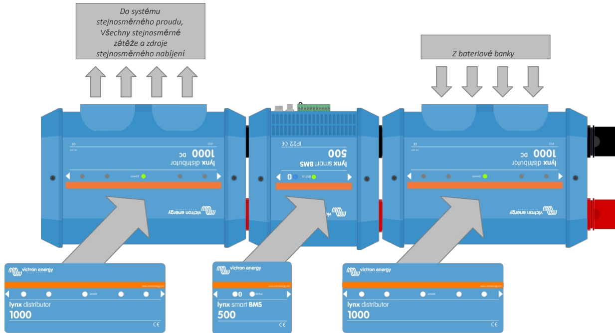
Příklad modulů Lynx namontovaných vzhůru nohama: baterie se připojují na pravou stranu, všechny zátěže a nabíječky se připojují na levou stranu a nalepí se nálepky vzhůru nohama.
