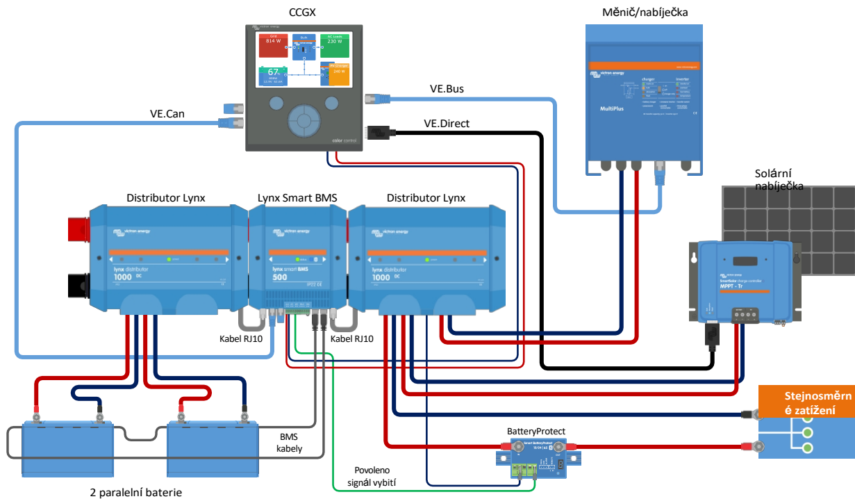
System s lithiovými bateriemi, Lynx Smart BMS a dvěma Lynx Distributory
