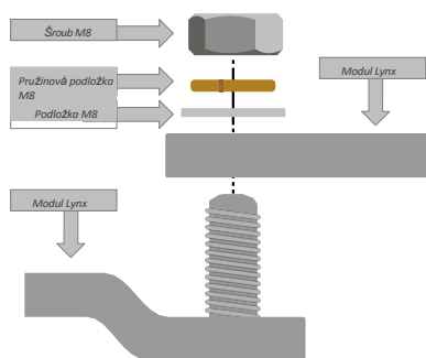
Obrázek 3. Pořadí připojení při připojení dvou modulů Lynx
