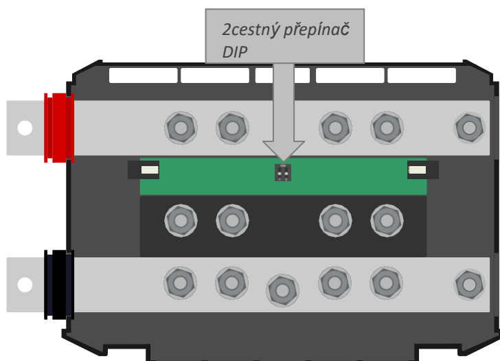
Obrázek 5. Umístění dvoucestného přepínače DIP distributora Lynx
